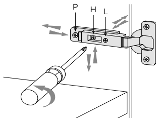
Réglage de la profondeur aisé par vis sans fin filetée +3/-2 mm
