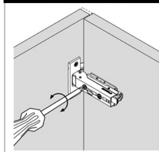
Réglage latéral avec limitation de la butée de +/-2 mm
