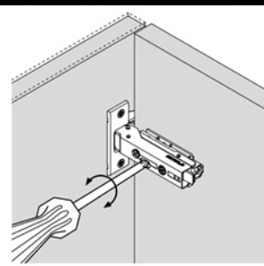
Réglage en hauteur par plaque de montage +/-2 mm
