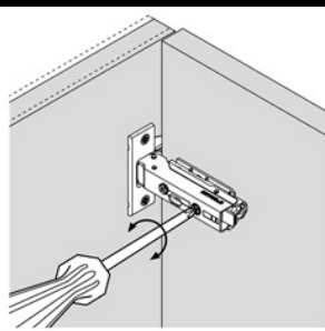
Réglage de la profondeur aisé par vis sans fin filetée +3/-2 mm
